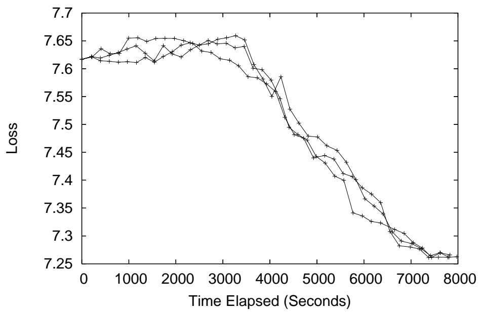
OLA-GD: Matchbox
